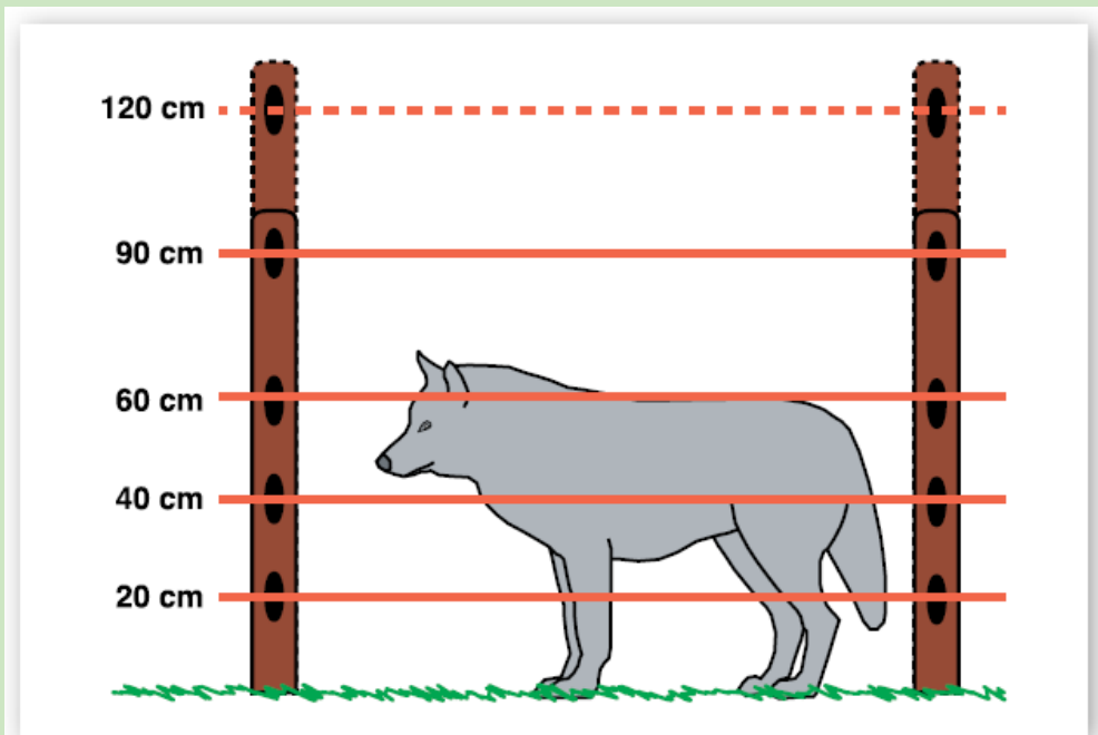
Abbildung 7: Grundaufbau Wolfsabwehrzaun (© G. Herkert)
